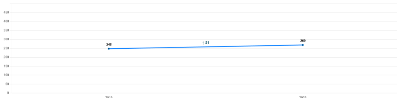
Comparación con establecimientos de similar GSE
